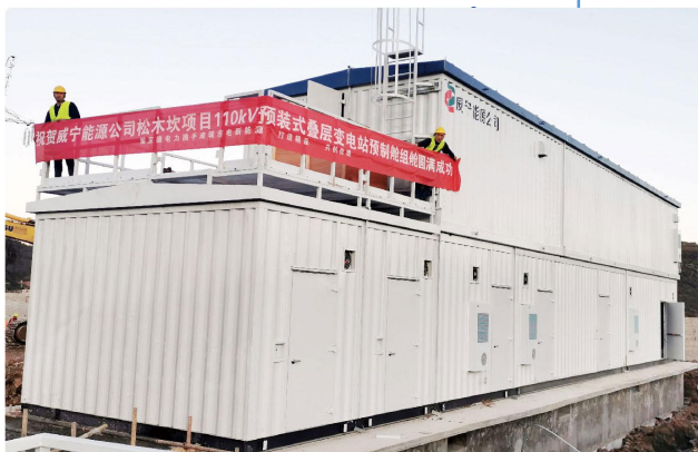
2019年11月 贵州省威宁县 麻乍松木坎110kV升压站项目
