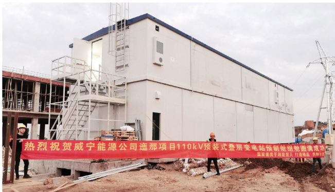
2019年11月 贵州省威宁县 迤那110kV装配式集成升压站
